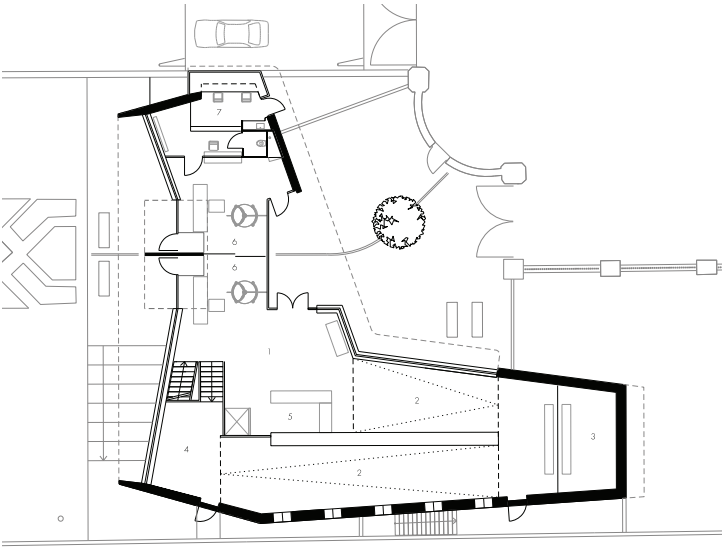
Grundriss Erdgeschoss
