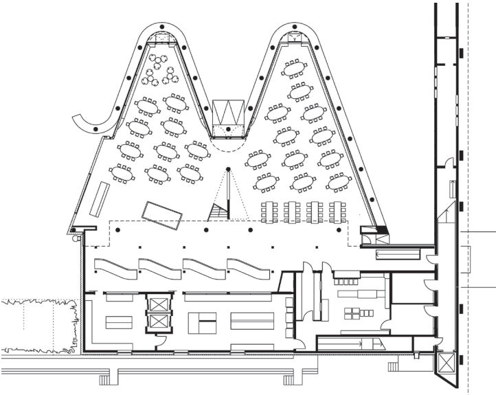
Grundriss Erdgeschoss
